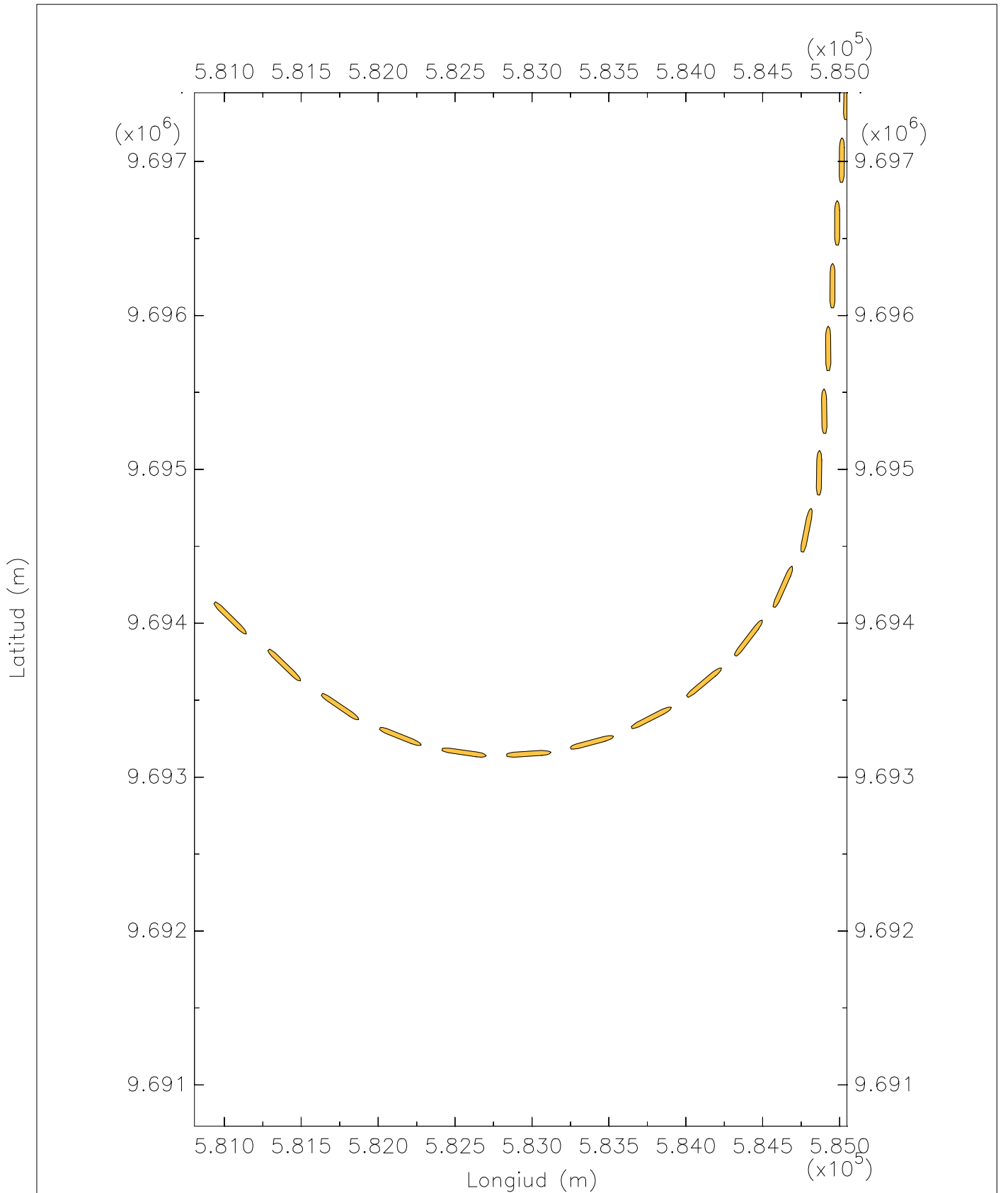
Z1T2 Trayectoria del barco portacontenedores panamax
