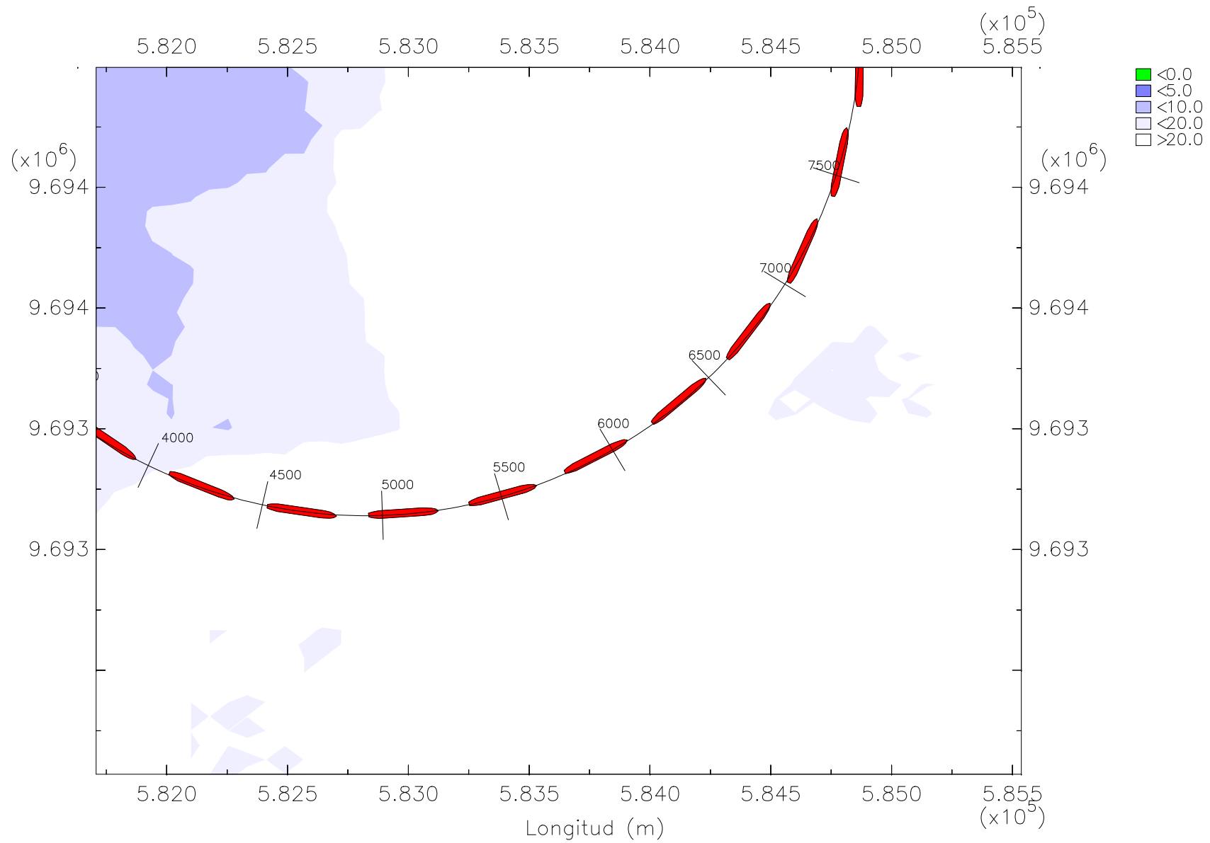
Z1T2 Trayectoria del barco portacontenedores panamax con profundidad
